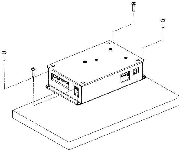
Abb.1 Montage Leistungsteil
