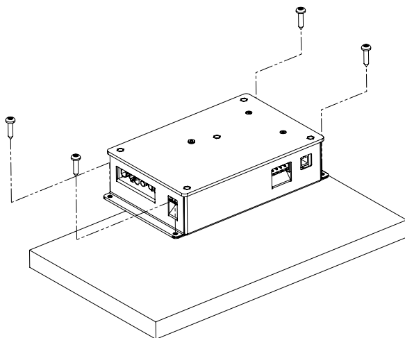
Obr. 1 Montáž výkonového dílu
