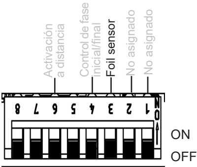
Fig. 12: Sensor de lámina
