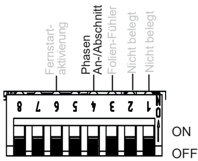
Abb. 17: Phase An-/Abschnitt
