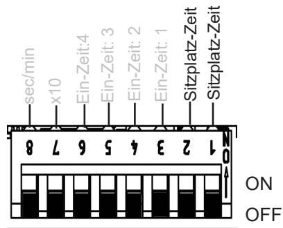
Abb. 13:Sitzplatz-Zeit
