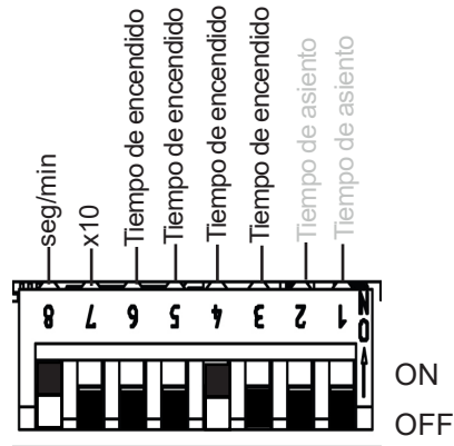
Fig. 15: Ejemplo de tiempo de encendido
