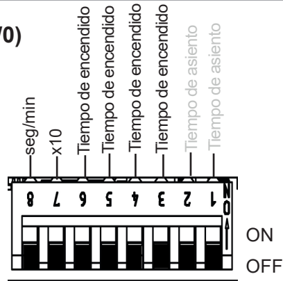
Fig. 14: Tiempo de encendido
