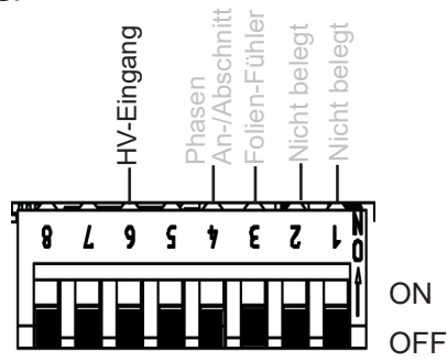
Abb. 18: HV-Eingang
