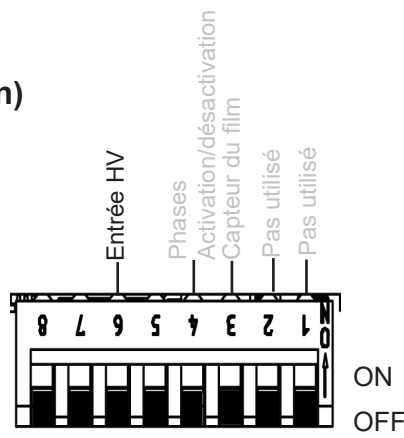
Fig. 18 : Entrée HV
