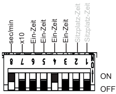
Abb. 15: Beispiel Ein-Zeit
