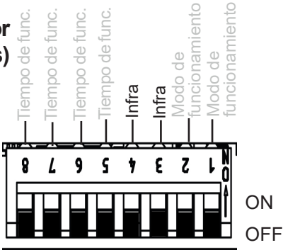
Fig. 10: Modo de funcionamiento Infra
