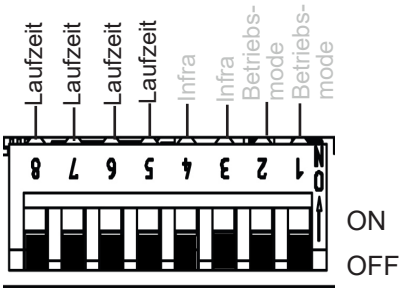
Abb. 11: Laufzeit
