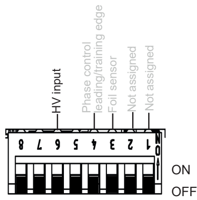
Fig. 18: HV input
