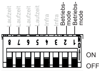
Abb. 9: Betriebsmodus
