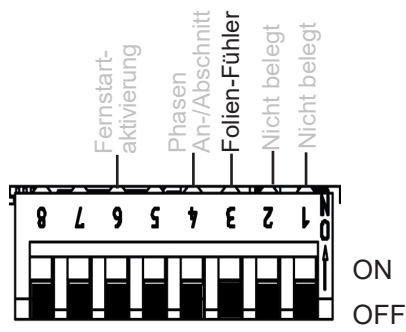
Abb. 12: Folienfühler
