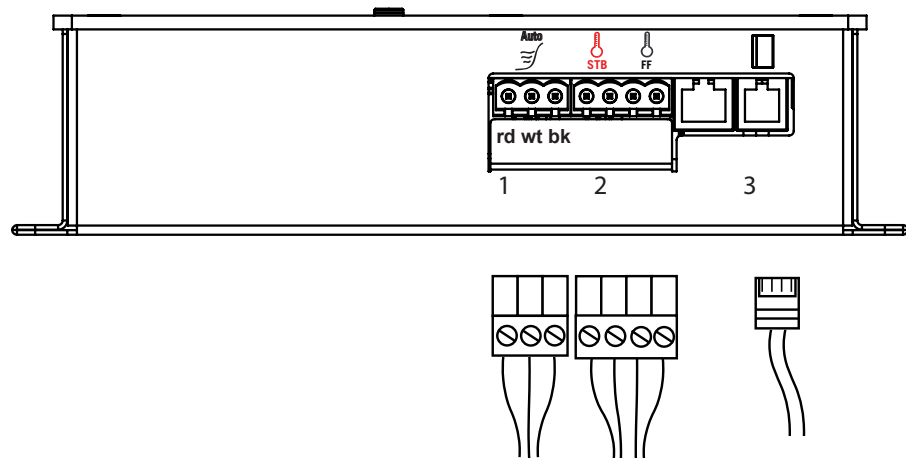
Fig. 6: Área de conexión para sensor/módulo de mando/sensor de asiento
