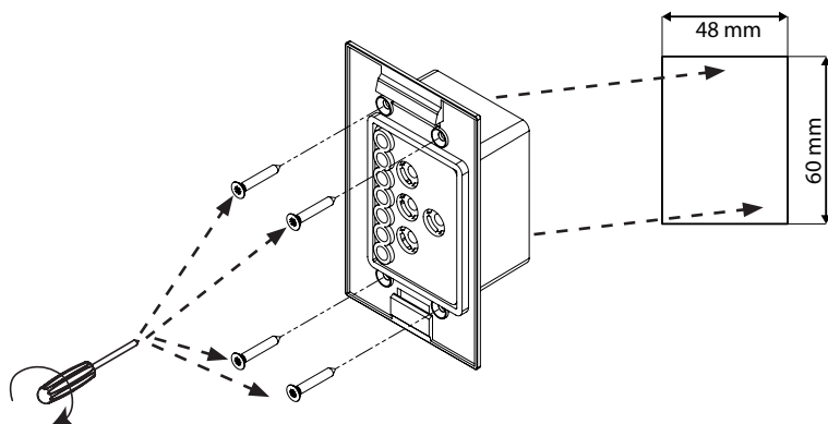
Obr. 3 Montáž ovladače
